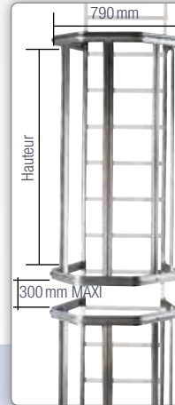
CRINOLINE STANDARD (Échelle non fournie avec la crinoline standard). Hauteur 0,62 à 1,46 m, tous les 28 cm.
